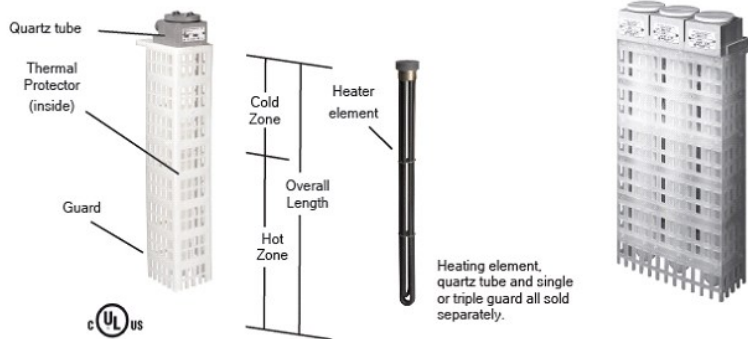
QM 系列石英加熱器合金屬元件
