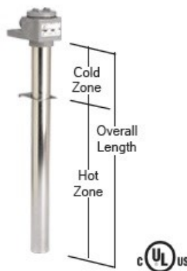
P, F, S and T 系列直立單管金屬加熱器
